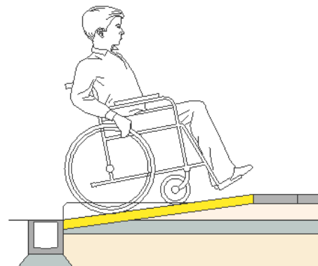
Pendenza 4-5%
